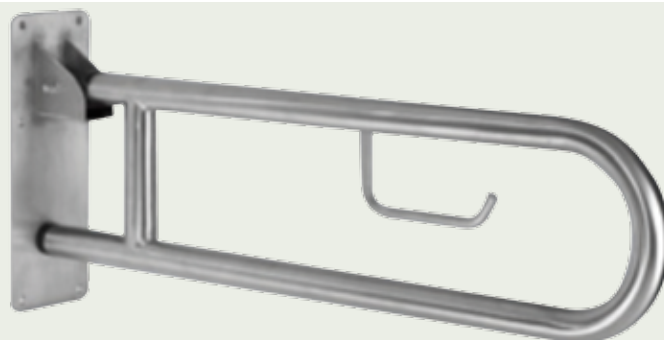
▲ Ref. JP00500 Barra abatible de acero inox. AISI 304 satinado con portarrollos. Medidas: 740 x 300 H x 90º
